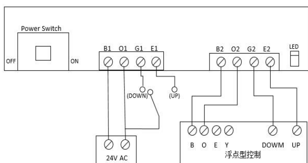
断电后执行器轴向上运行
