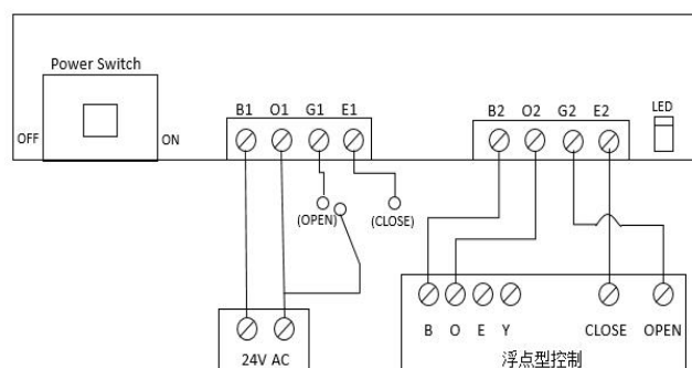
断电后球阀关闭
