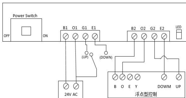
断电后执行器轴向下运行
